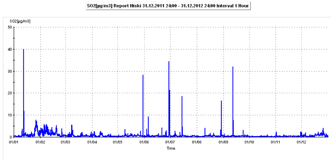
Rikkidioksidi (SO 2 ) tuntiarvot Hiskinmäki 2012, raja-arvo 350 µg/m 3
